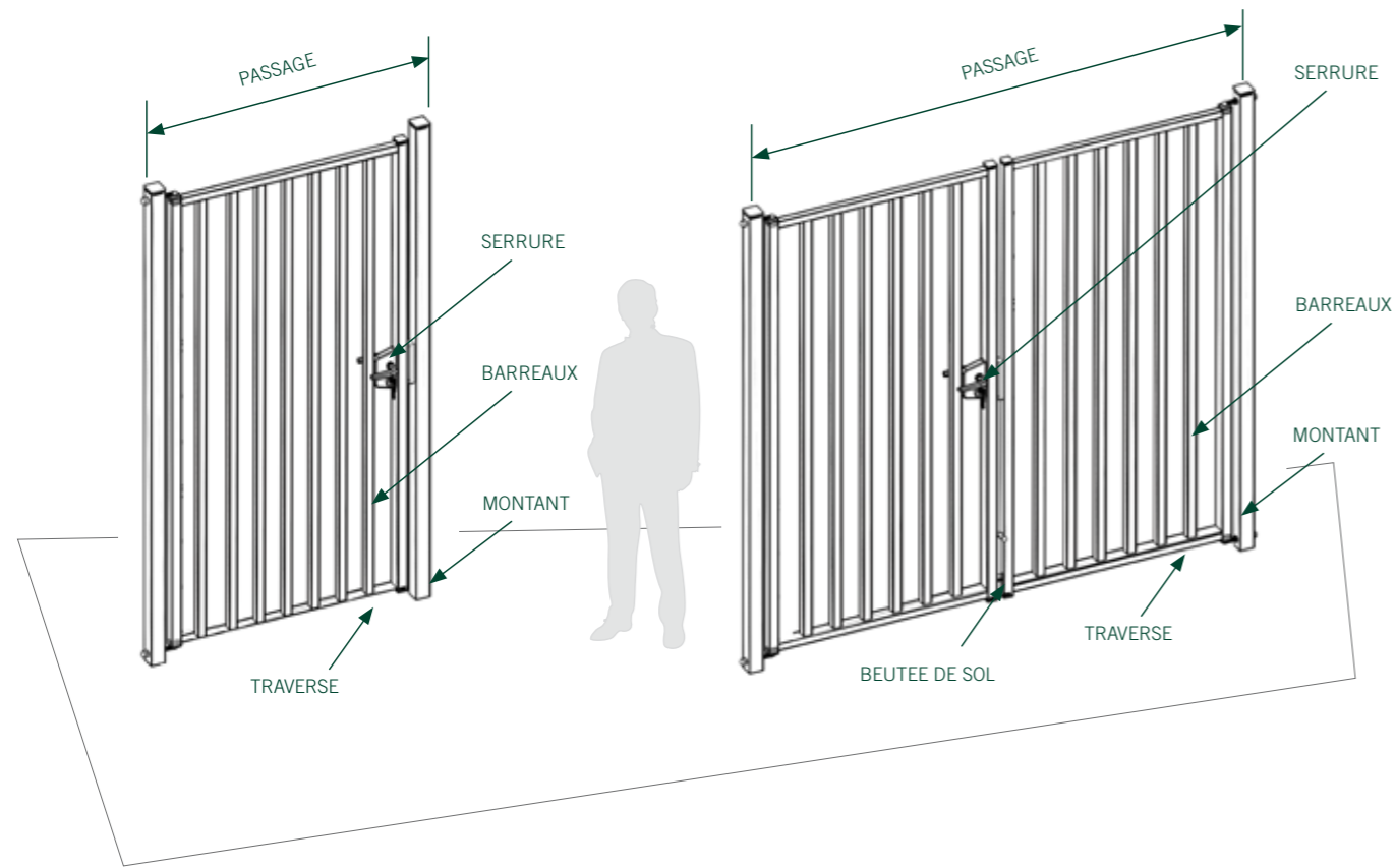
PORTAIL À UN VANTAIL Ouverture intérieure droite (standard)
